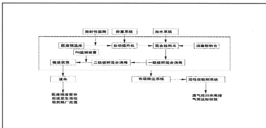
(干式碱性化学消毒工艺流程图)
